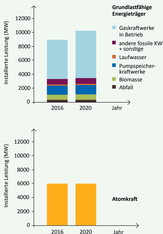
Grafik 2: Vergleich der Kapazität von grundlastfähigen Kraftwerken und Atomkraftwerken (in Belgien) Daten: Entso-e 2020
